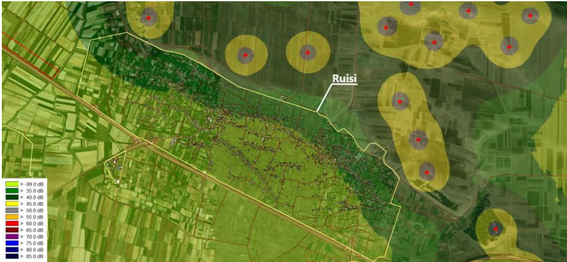
სურათი 3-2 ხმაურის მოდელირების სქემების ნიმუში: ხმაურის გავრცელება სოფ. რუსის მიდამოებში - ტურბინის სიმაღლე შეადგენს 150 მ-ს.
